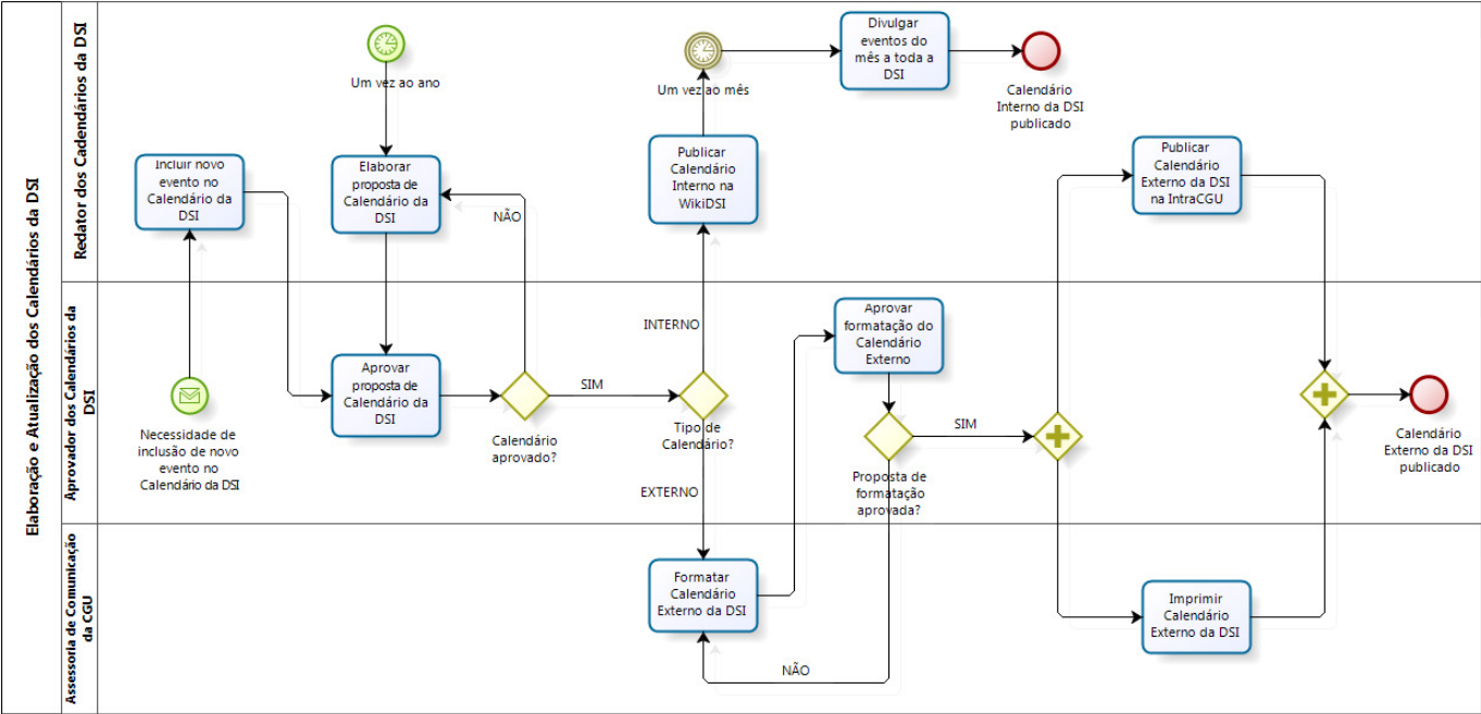
Diagrama BPMN do Processo de Elaboração e Atualização dos Calendários da DSI
